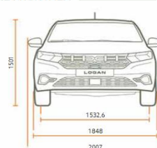
VEDERE FRONTALĂ
